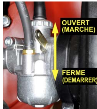
Levier de l'étrangleur
