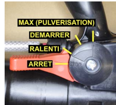
Levier de la manette
